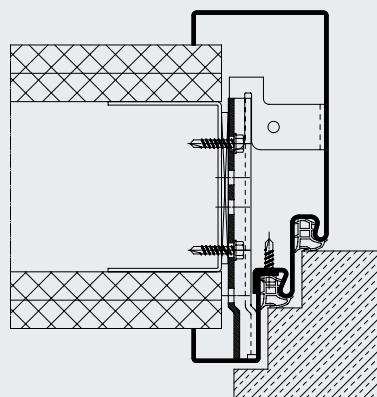
2-részes acéltok, dupla falcolt ajtóhoz
