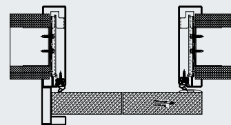
Fal előtt futó tolóajtó-tok, szorosan záródó
